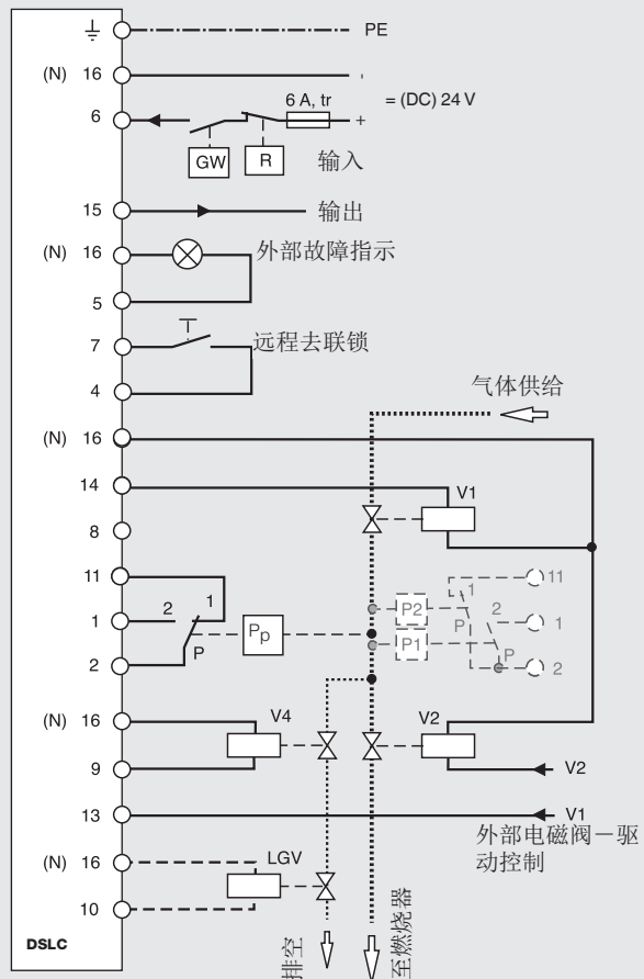
用于直接控制阀门V1, V2的DSLCL接线图 (对应原理示意图4)
