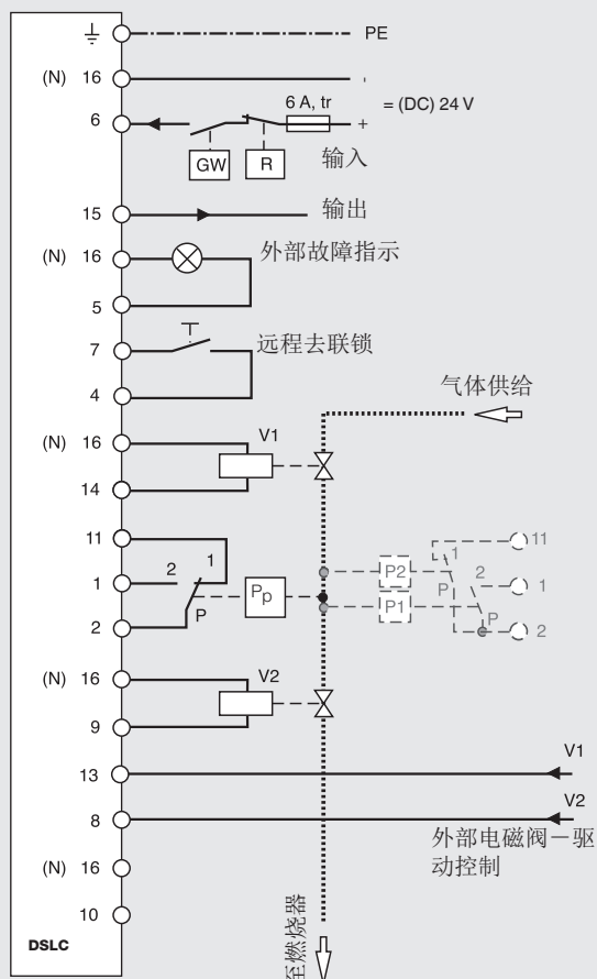
用于带辅助阀V4或LGV直接控制阀门V1的DSLCL接线图 (对应原理示意图3)
