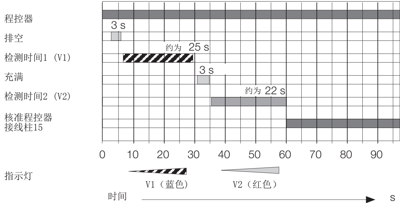
密封检测装置DSLC px Vx的结构
